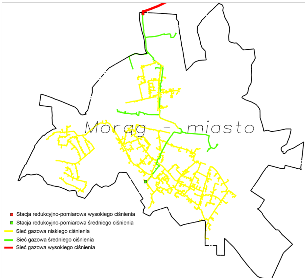
Rysunek 5. Schemat infrastruktury gazowniczej – miasto Morąg
