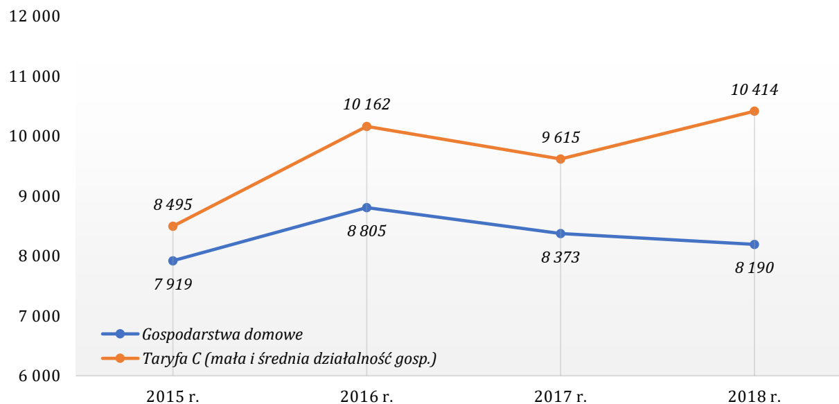
Wykres 32. Zużycie energii elektrycznej na terenie miasta Morąg w latach 2015-2018 przez gospodarstwa domowe oraz małe i średnie podmioty gospodarcze (handlowo-usługowe) [MWh]
