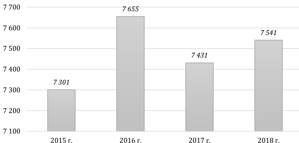
Wykres 10. Zużycie mialu węglowego w Kotłowni Rejonowej w latach 2015-2018 [Mg]
