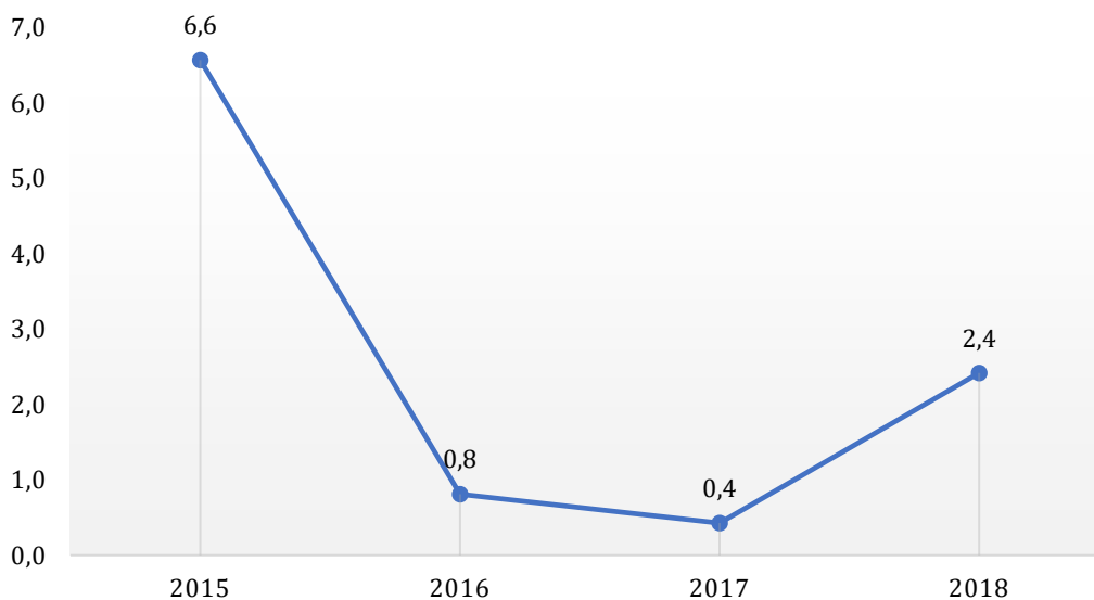
Wykres 23. Wielkość emisji pyłu z Kotłowni Rejonowej w latach 2015-2018 [Mg]
