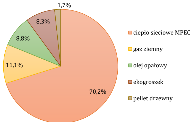
Wykres 19. Udział poszczególnych nośników ciepła wykorzystywanych na cele c.o. w budynkach oświatowych na terenie gminy (pod kątem ogrzewanej powierzchni)
