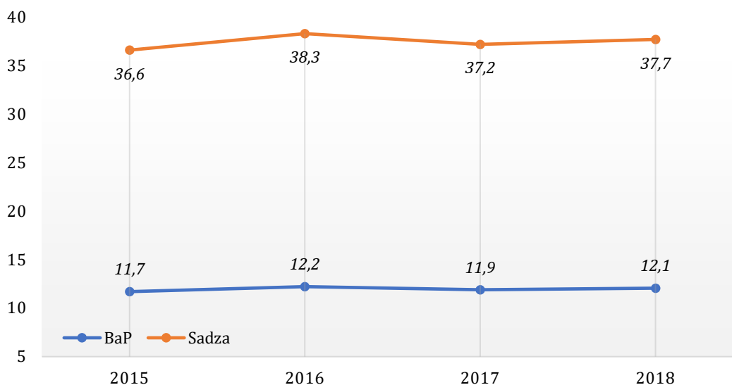
Wykres 22. Wielkość emisji B(a)P oraz sadzy z Kotłowni Rejonowej w latach 2015-18 [kg]
