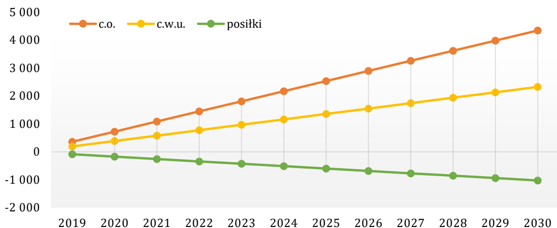
Wykres 26. Przewidywana zmiana zapotrzebowania na ciepło w sektorze mieszkalnictwa związana z oddawaniem do użytkowania nowych budynków mieszkalnych oraz zmianą liczby ludności - MIASTO MORĄG [GJ]
