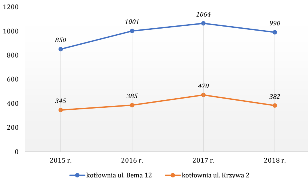
Wykres 13. Produkcja ciepła w kotłowniach lokalnych w latach 2015-2018 [GJ]
