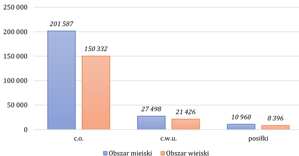
Wykres 18. Aktualne szacunkowe zapotrzebowanie na ciepło w sektorze budynków mieszkalnych na terenie gminy [GJ]
