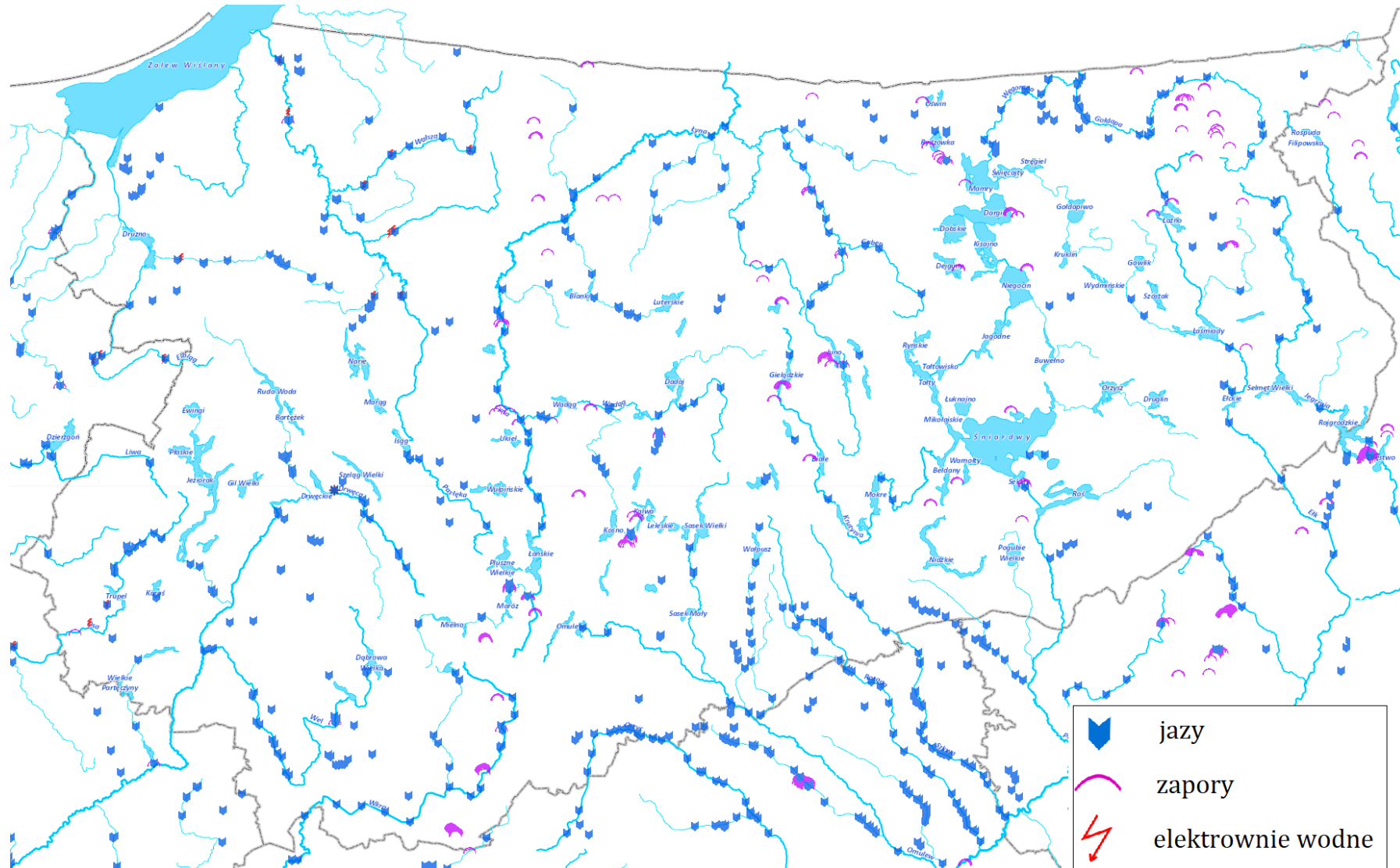
Rysunek 11. Lokalizacja jazów oraz zapór wodnych na terenie województwa warmińsko-mazurskiego jako potencjalnych miejsc lokalizacji elektrowni wodnych
