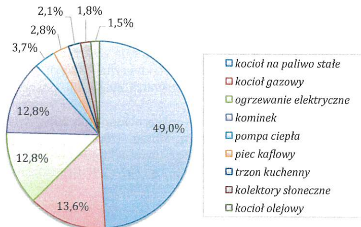
Wykres 16. Struktura indywidualnych urządzeń grzewczych stosowanych na terenie gminy
