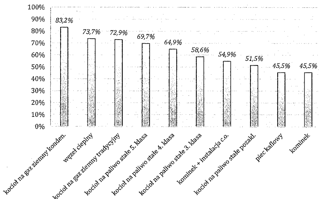
Wykres 15. Orientacyjne całkowite sprawności systemów ogrzewania w zależności od stosowanego źródła ciepła Źródło: opracowanie własne
