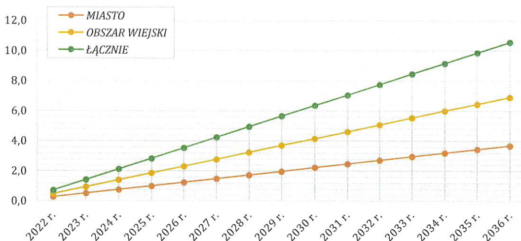
Wykres 37. Przewidywany przyrost zapotrzebowania na moc elektryczną w sektorze gospodarstw domowych na terenie Gminy Morąg w perspektywie do 2036 r. [MW]
