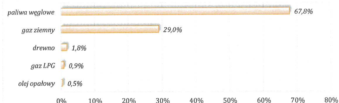
Wykres 19. Udział poszczególnych nośników energii w zużyciu ciepła przez podmioty gospodarcze prowadzące działalność na terenie Gminy Morąg
