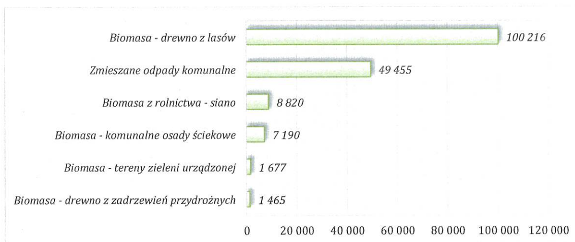
Wykres 43. Teoretyczny roczny potencjał energetyczny zasobów biomasy stałej na terenie Gminy Morąg [GJ]
