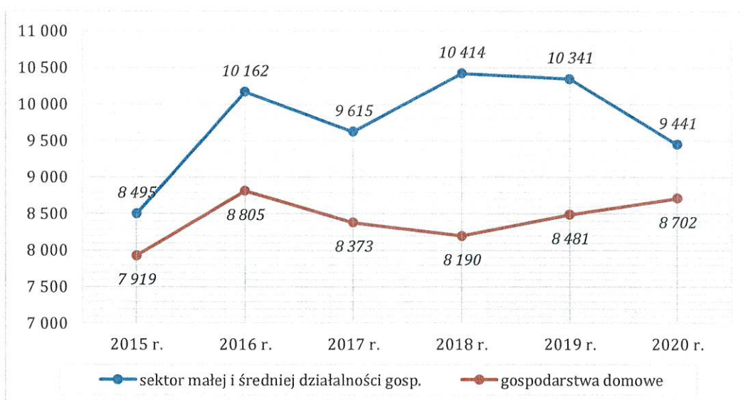
Wykres 34. Zużycie energii elektrycznej na terenie miasta Morąg w latach 2015-2020 (gospodarstwa domowe oraz sektor małej i średniej działalności gospodarczej) [MWh] Źródło: ENERGA-OPERATOR S.A.
