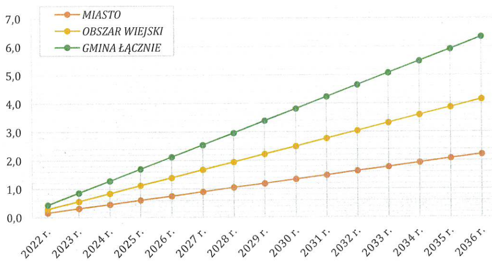
Wykres 29. Prognozowany przyrost zapotrzebowania na moc cieplną (c.o.) w sektorze mieszkalnictwa na terenie Gminy Morąg związany z oddawaniem do użytkowania nowych budynków mieszkalnych w perspektywie do 2036 r. [MW]
